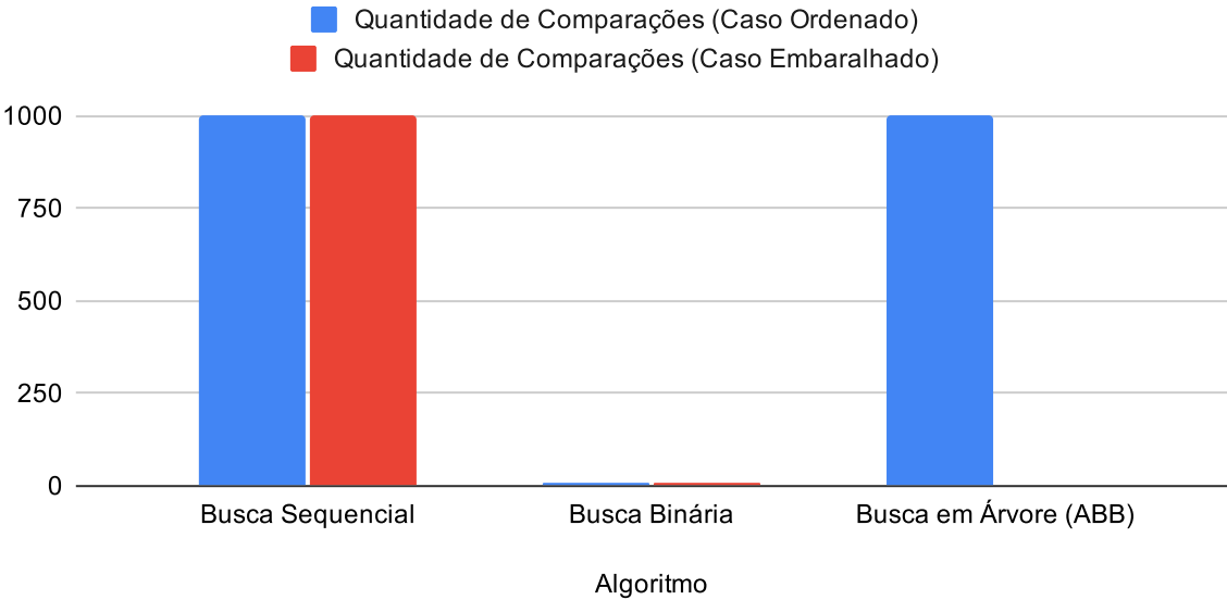
Quantidade de Comparações (Caso Ordenado) e Quantidade de Comparações (Caso Embaralhado)
